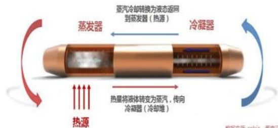
熱管散熱示意圖
