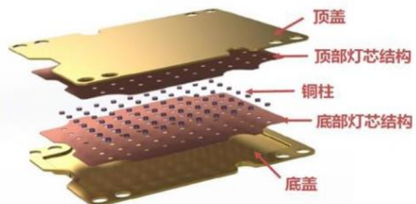
VC中間是氣室結構(即燈芯)
